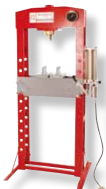
WP 30H WERKSTATTPRESSE / SHOP PRESS
