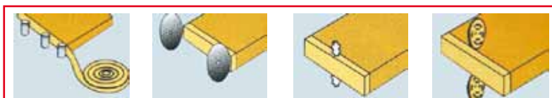
Kleben glueing Kantenendanschnitt end cutting Doppelfrässaggregat finishing R side Polieraggregat buffing
