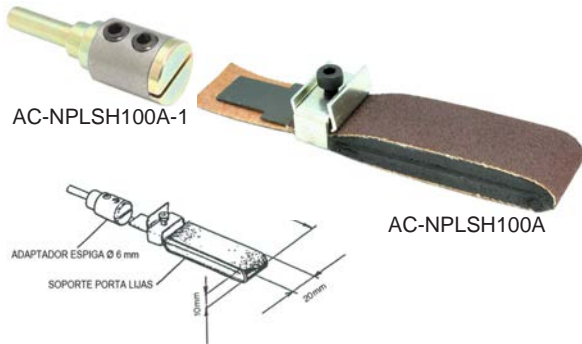
AC-NPLSH100A-1 ADAPTADOR ESPIGA Ø 6 mm AC-NPLSH100A SOPORTE PORTA LIJAS
