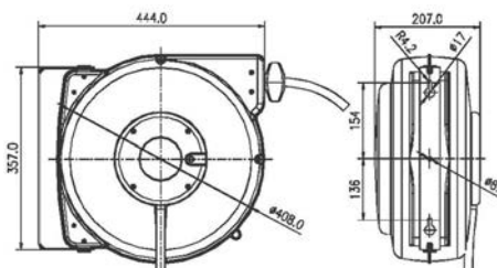
HR-CR625201SG 230 V - 20 metros ENROLLADOR DE ALTA RESISTENCIA CON GRANDES LONGITUDES DE CABLE
